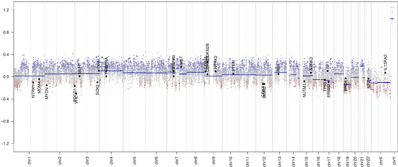
208416840105_R02C01_1
