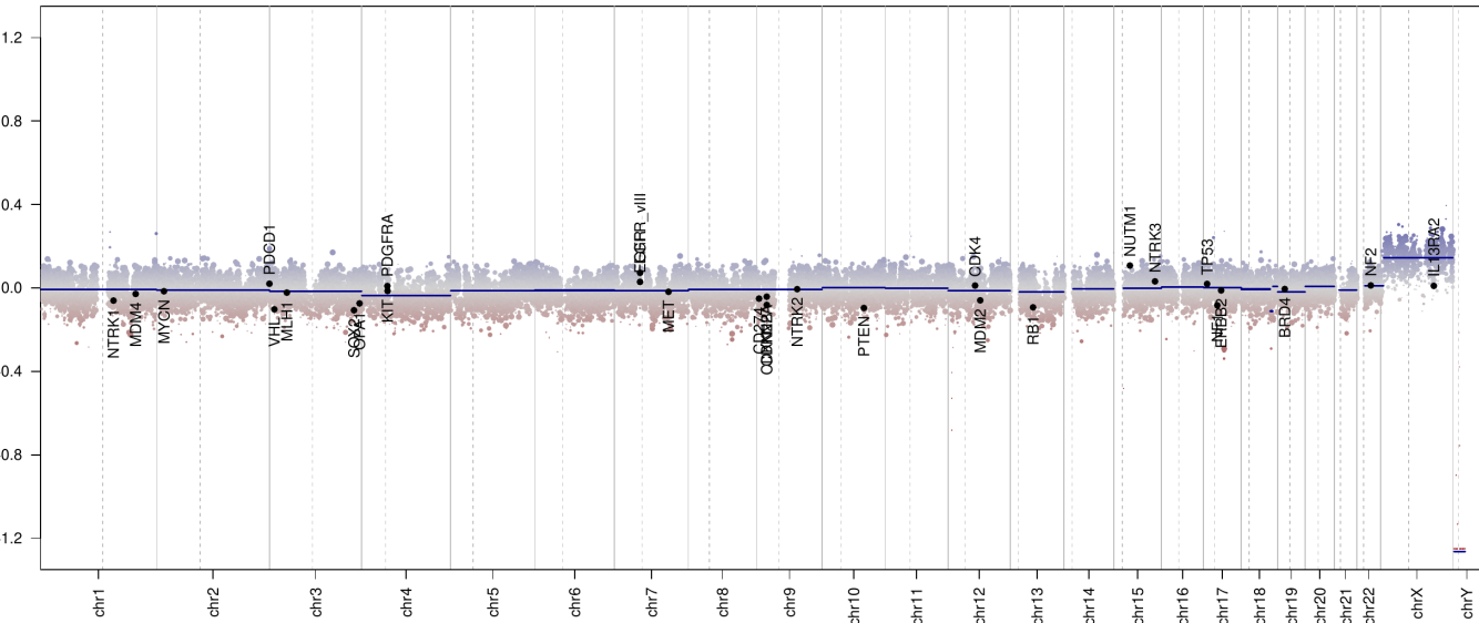
209717470157_R02C01
