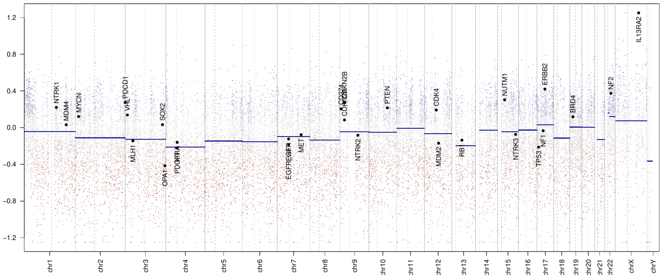
206375080148_R08C01
