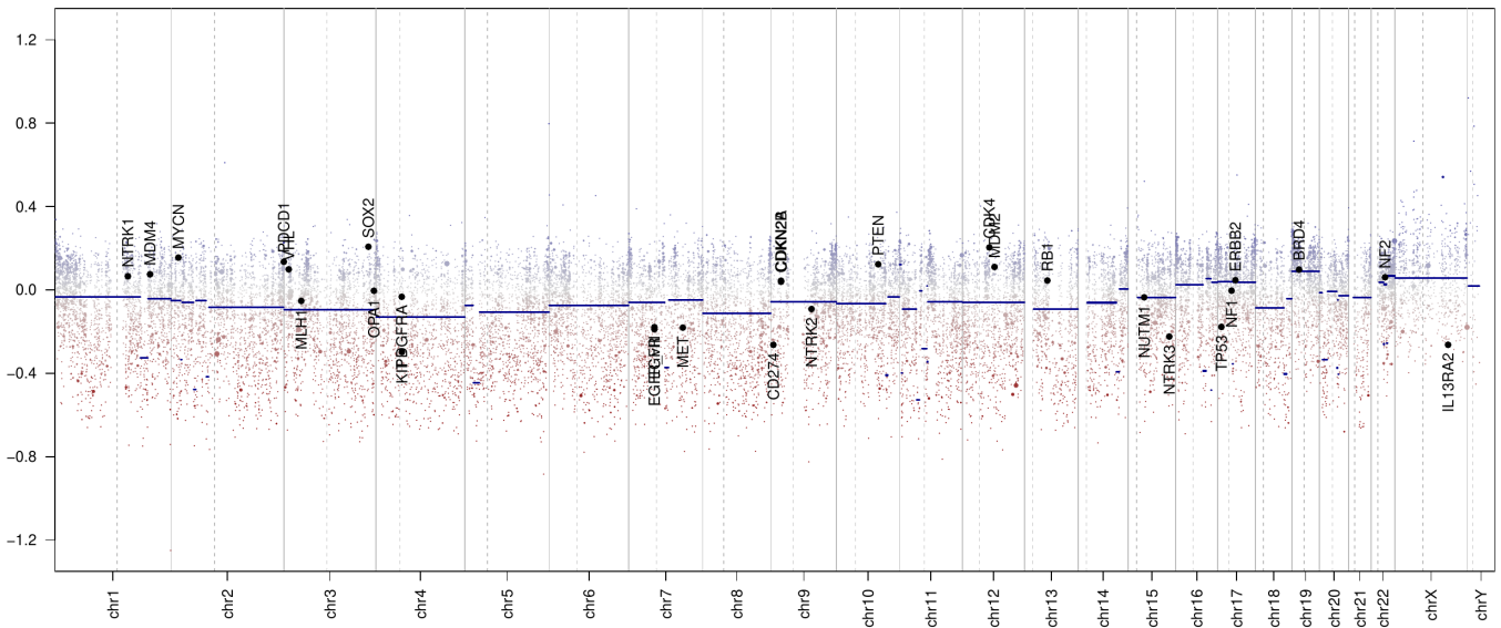
208356120158_R08C01
