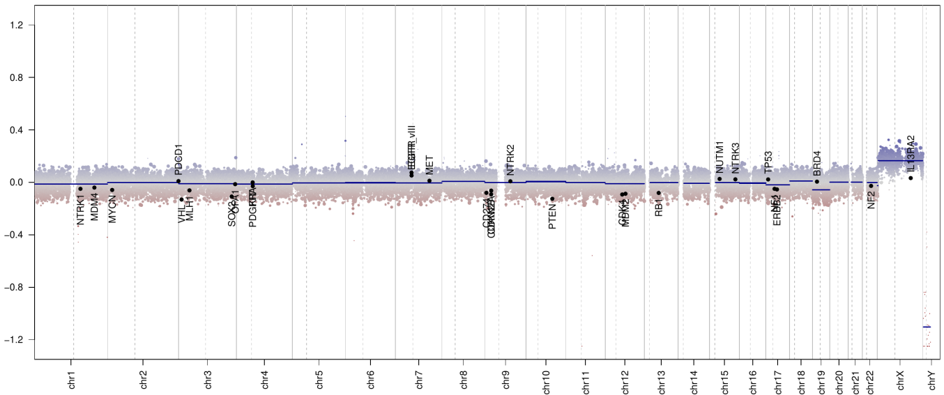
208654660117_R02C01
